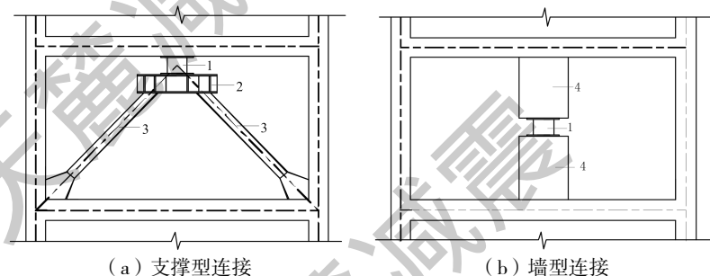
图 8.1.1 连接示意图
