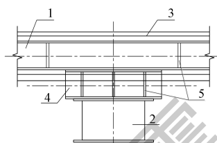
(I) 焊接连接
