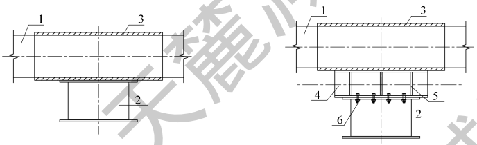
(I) 焊接连接
