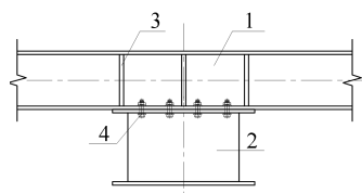
(II) 螺栓连接
