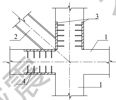
图 A.0.1-2 钢支撑与现浇混凝土框架节点域连接构造
