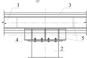
(II) 螺栓连接
