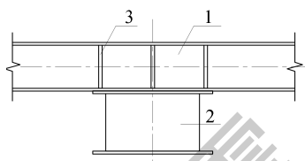
(I) 焊接连接
